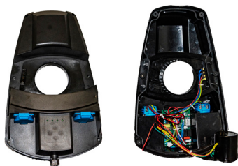
Låg el-del med printkort / Lock el-del med kretskort Art.nr. 41910
